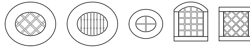
Esempi di occhi e finestre sopra luce con cornice in pietra o con cornice in muratura e intonaco con grate in ferro a disegni semplici
