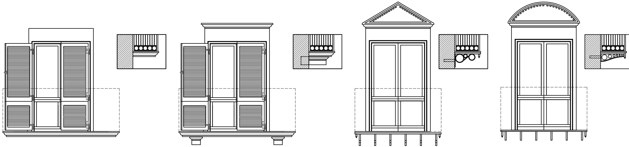
Balcone in c.a. o pietra con modanature sagomate Porta - finestra in legno con cornice
