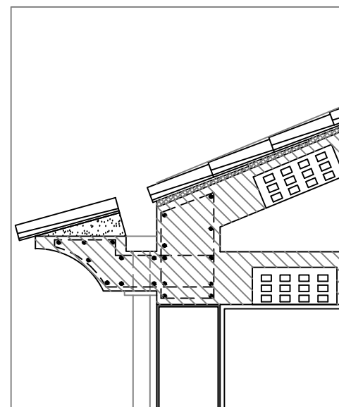
Cornicione in aggetto eseguito in contiguità con il cordolo in c.a.
