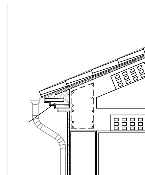
Cornicione in aggetto eseguito con tre file di coppi (romanella)
