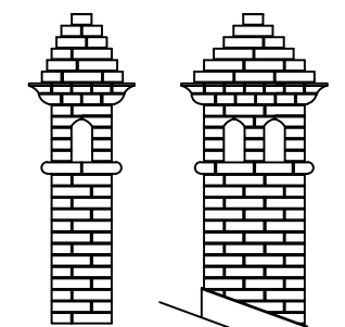
Esempi di comignoli in mattoni a disegno semplice
